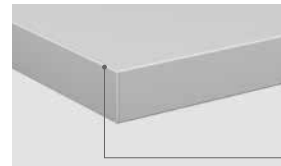
PUR Schmelzkleber
